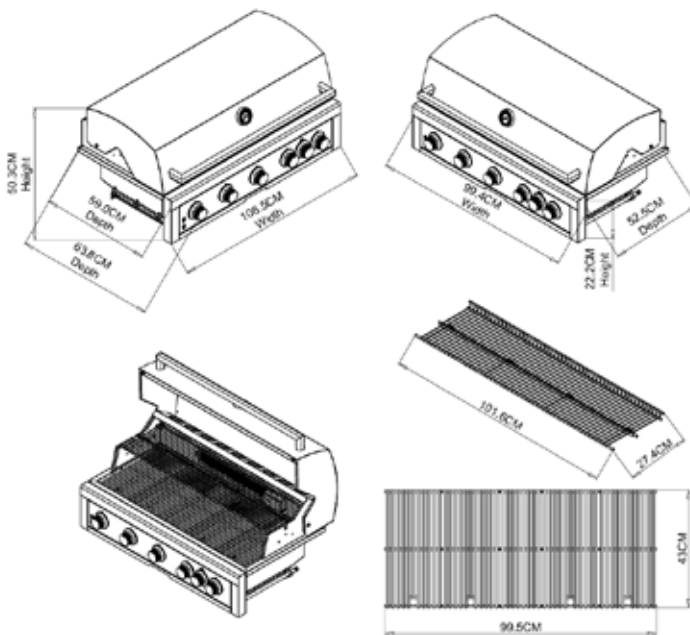
MODELO ST-G5B-IR
