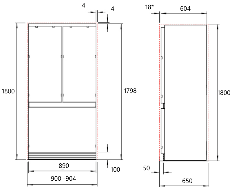
Medidas sin paneles frontales
